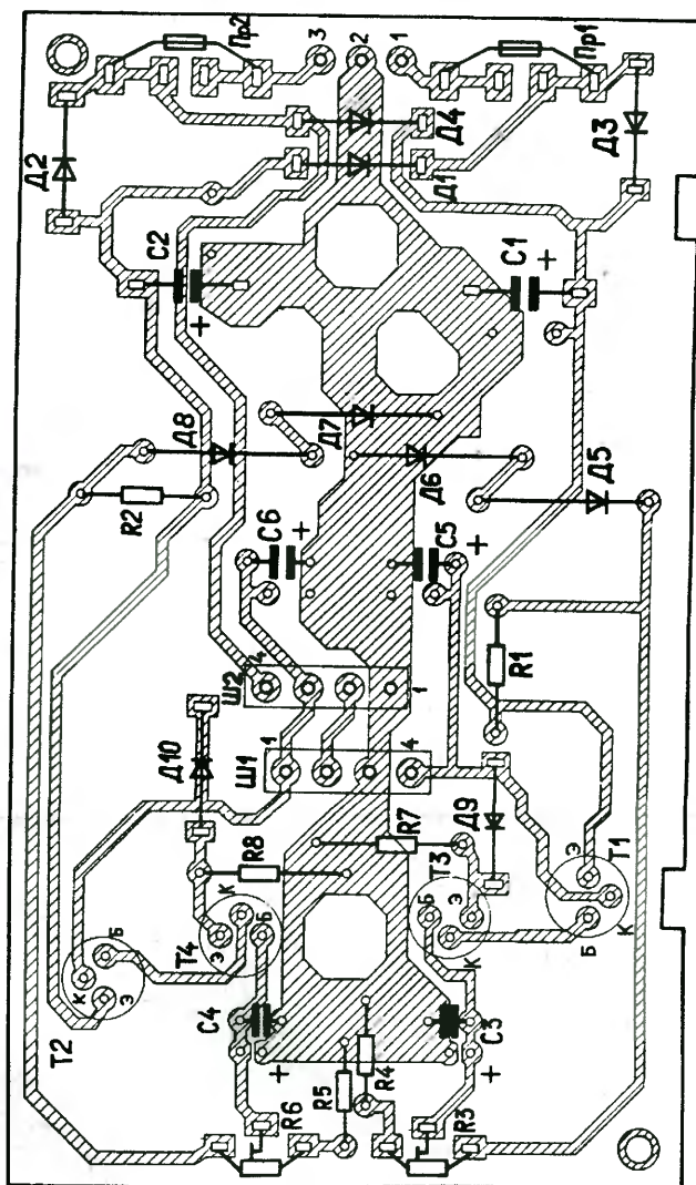
ПЛАТА СТАБИЛИЗАТОРА (У2)
