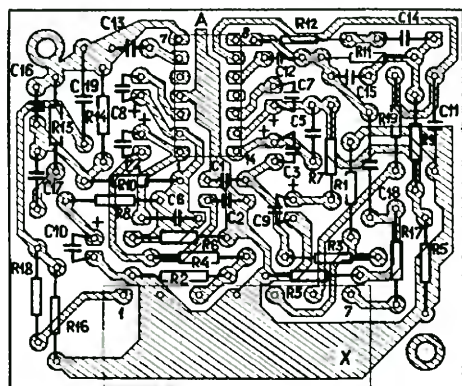
ПЛАТА УПЗ-15 (У3)
