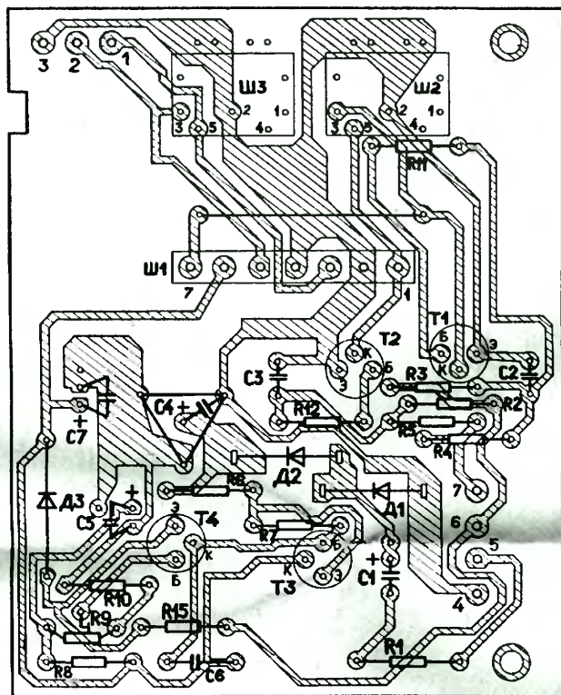
ПЛАТА УПЗ-15 (У3)
